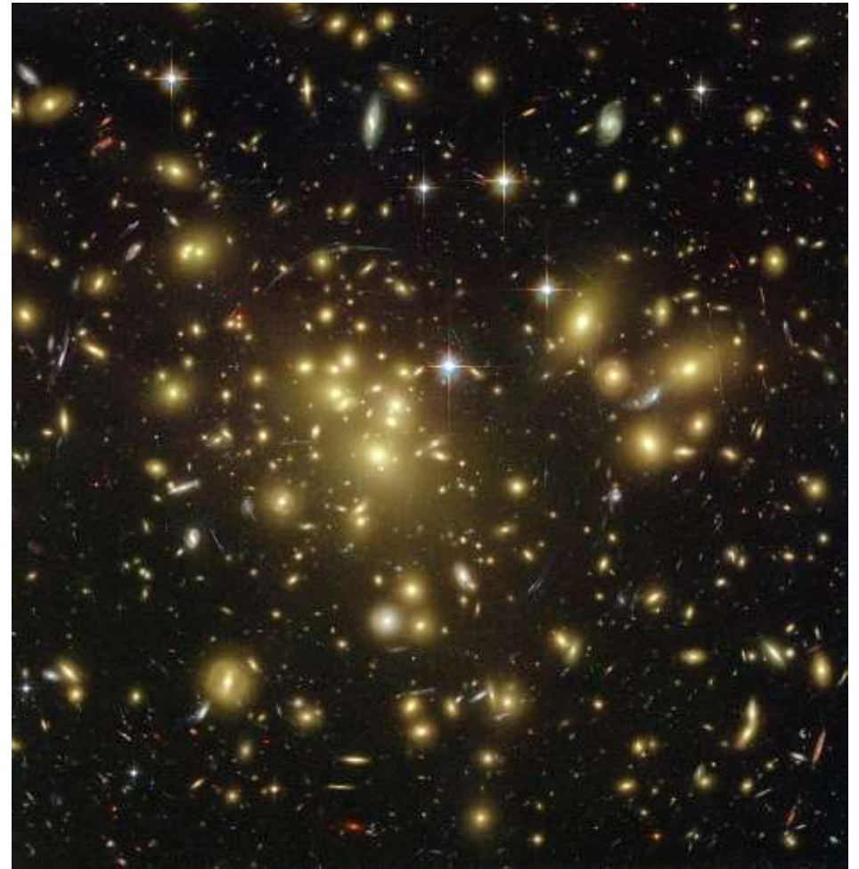
Le vertigineux amas de galaxies Abell 1689
