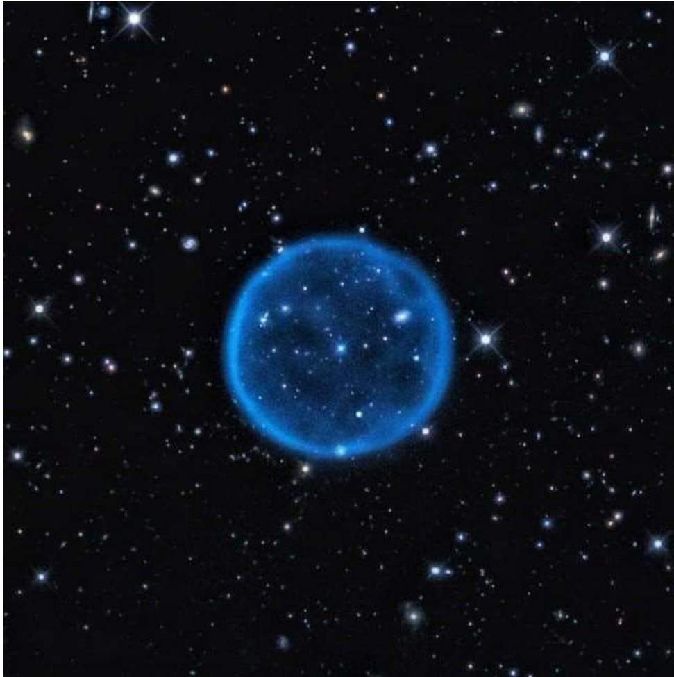
La très belle nébuleuse planétaire Abell 39
